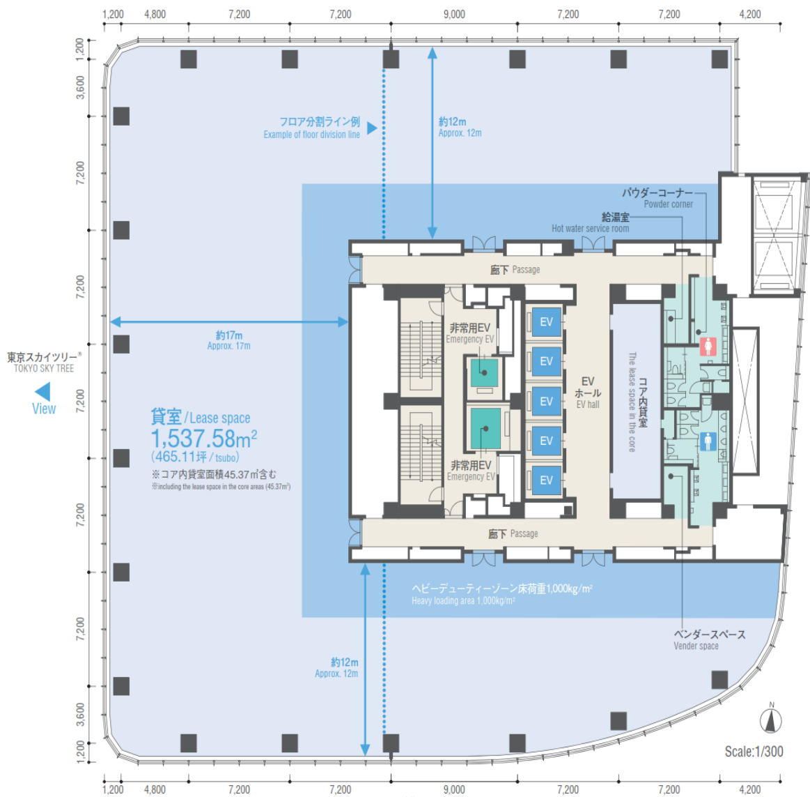
基準階平面図 (26F~29F) Standard floor plan (26F~29F)
